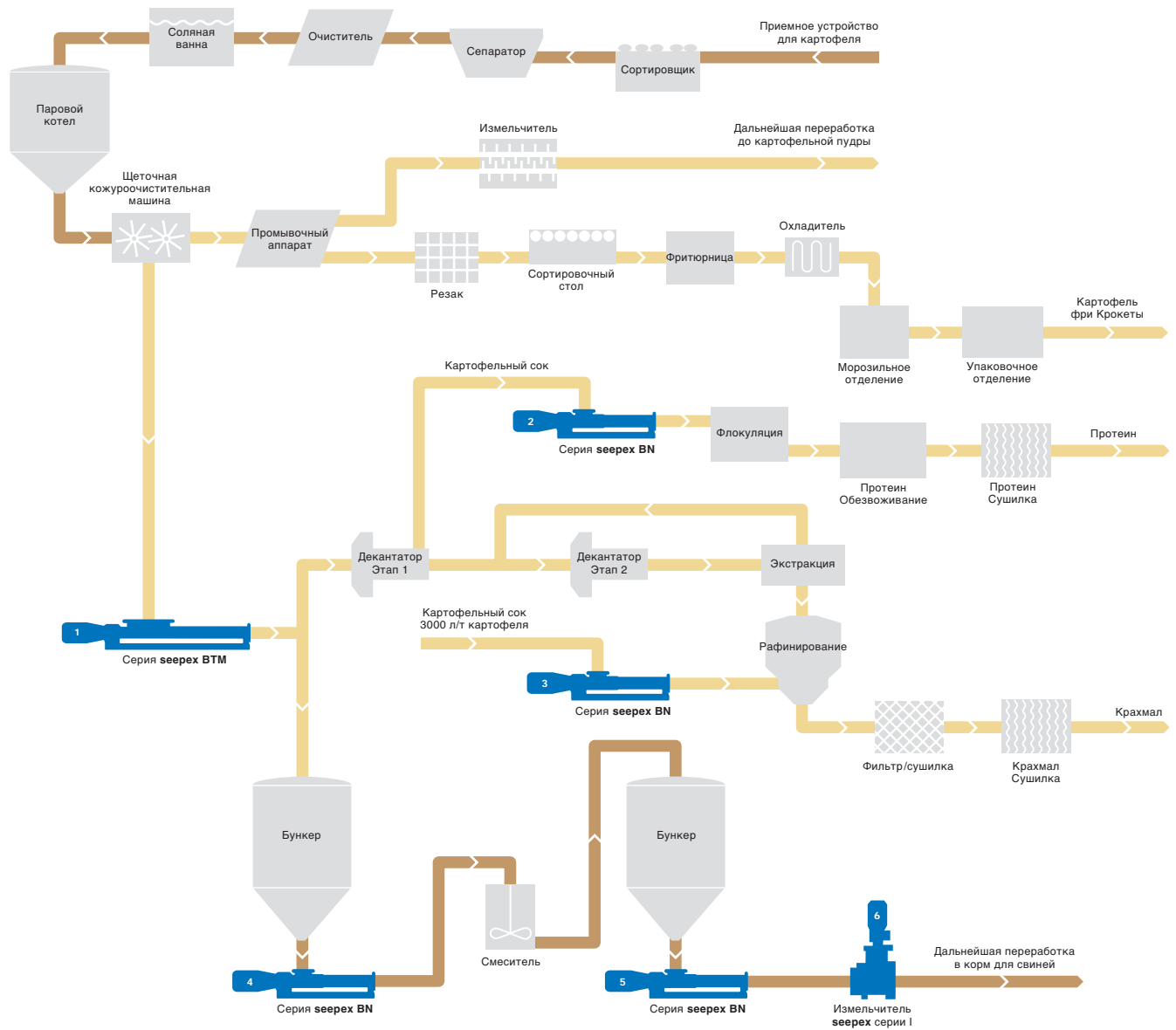
Технологический процесс переработки картофеля
